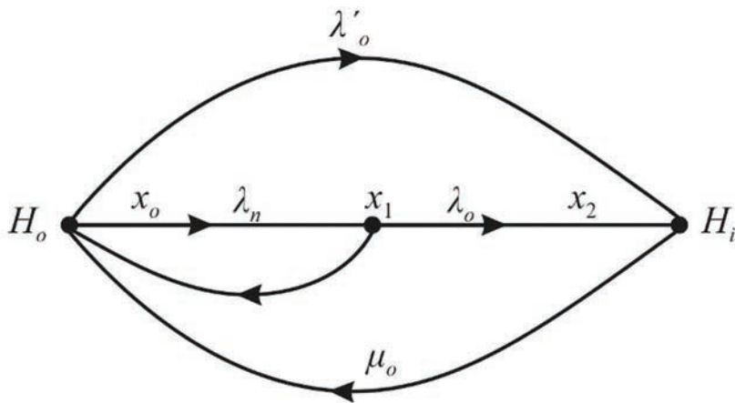
Рисунок 5 – Граф переходів трактора зі стану працездатності ( H_o ) у стан непрацездатності ( H_i ):
