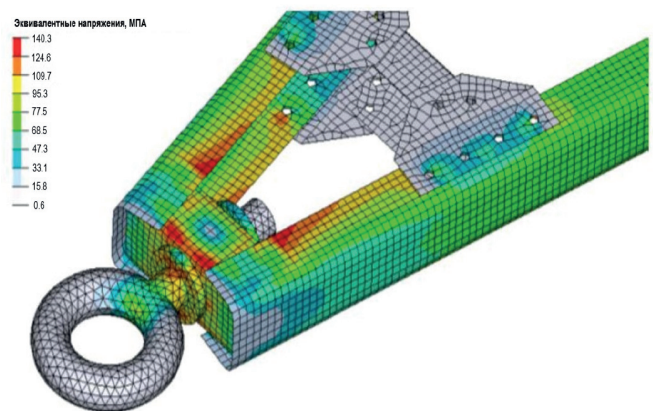
Рисунок 3 – Схема розподілення внутрішнього навантаження в кінцевій частині тягово-зчіпного пристрою причепа 2ПТС6
