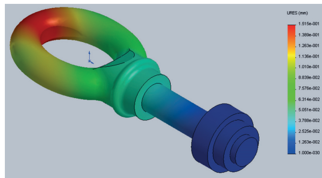
Рисунок 6 – Результати комп'ютерного розрахунку подовжень у зчіпній петлі
