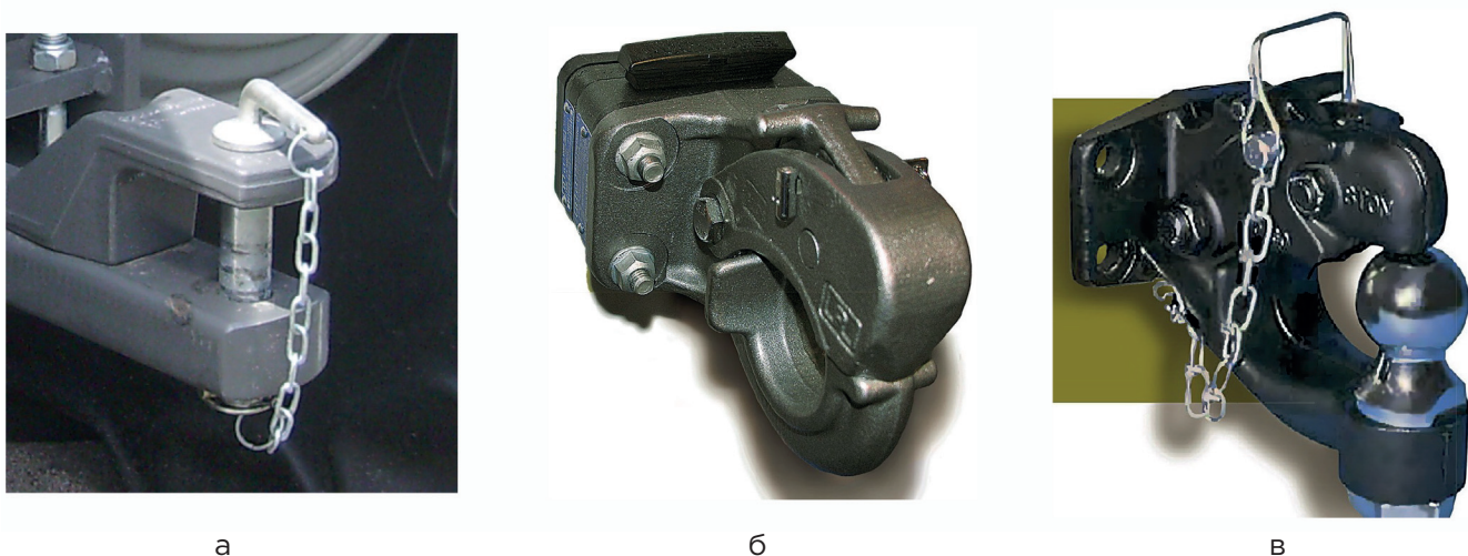
Рисунок 1 – Типи тягово-зчіпних пристроїв
