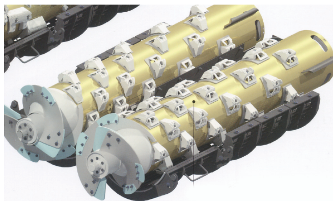
Рисунок 3 – Двуроторна система обмолоту комбайнів серії SR New Holland
