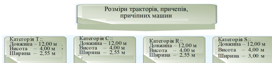
Рисунок 3 – Розміри сільськогосподарських та лісогосподарських транспортних засобів за їхніми категоріями
