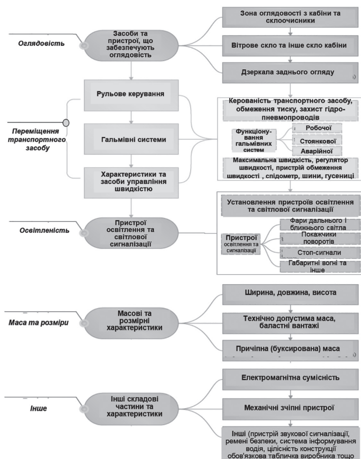
Рисунок 2 – Основні групи складових частин, систем, технічних вузлів і характеристик які визначають функційну безпеку сільськогосподарських та лісгосподарських транспортних засобів
