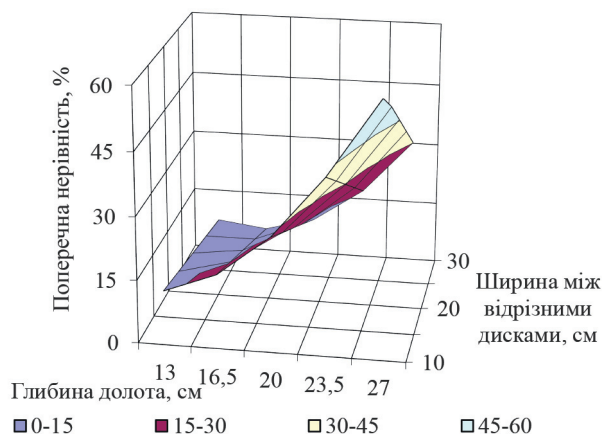
Рисунок 6 – Залежність поперечної нерівності від глибини обробітку долотом H та відстані між боковими відрізними дисками B , на швидкості руху МТА V = 7,5 км/год
