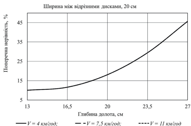
Рисунок 7 – Залежність поперечної нерівності від глибини обробітку долотом H за відстані між боковими відрізними дисками B = 20 см
