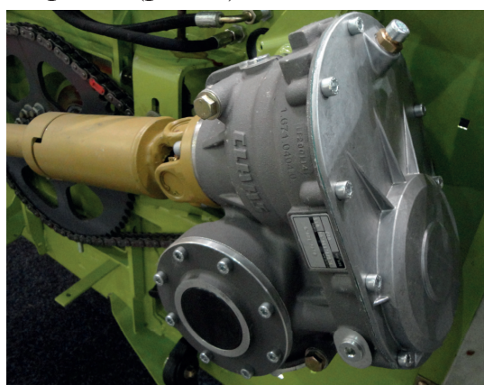
Рисунок 6 – Редуктор для приводу ножа широкозахватної жатки
