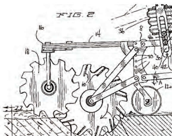
Рисунок 4 – Засіб і спосіб смугового обробітку ґрунту (Zone tillage tool and method) [Bauer, 2006]
