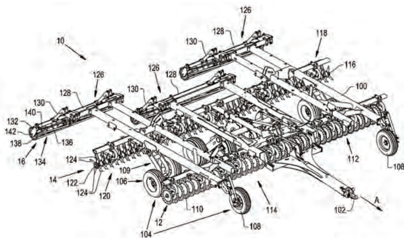
Рисунок 5 – Комбінований ґрунтообробний агрегат для вертикального обробітку й аерації ґрунту (Hybrid tillage implement for vertical tillage and aeration of soi) [Roberge & Hall, 2018]
