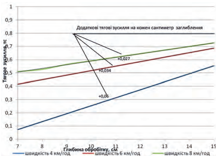
Рисунок 4 – Залежність тягового зусилля від глибини обробітку на різних швидкостях
