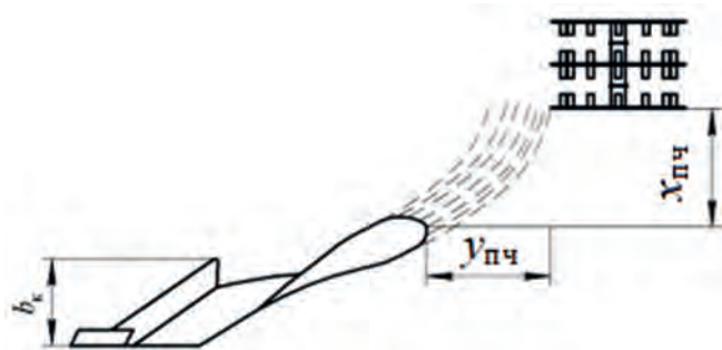
Рисунок 1 – Схема установки дополнительных почвообрабатывающих устройств относительно корпуса плуга
