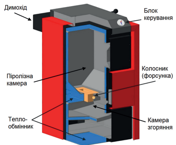
Рисунок 1 - Піролізний котел
